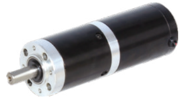
45JX永磁直行星减速电机 用于全自动割草机的行走电机
